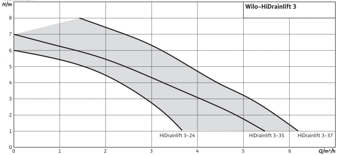
Kennlinien
